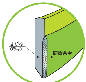
快適Z爪断面図
