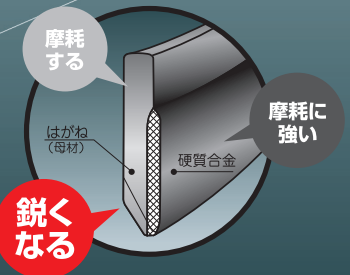
Z爪断面図
